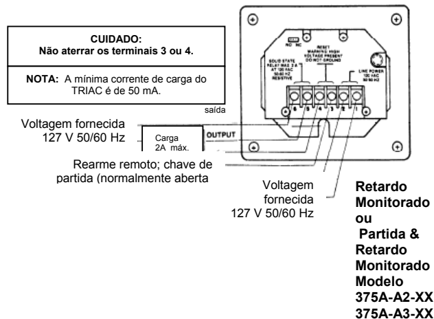
Figura 2b - Fiação externa para o Vibraswitch Modelo 375A
