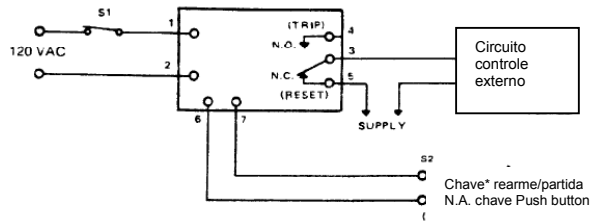
Vibraswitch com retardo na partida (Modelo 375A/376A-A1-XX)
